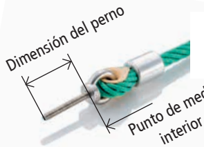
Anillo de acero inoxidable Art. No. 455B M8/M10/M12 con tornillo pegado galvanizado
